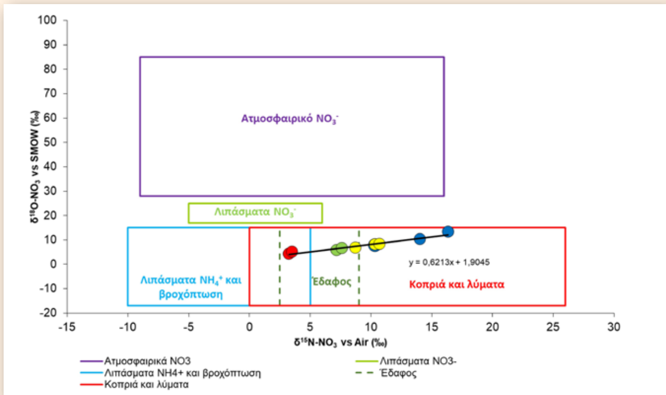
Σχήμα 2. Διάγραμμα συσχέτισης του \delta^{15}\text{N}-\text{NO}_3^- με το \delta^{18}\text{O}-\text{NO}_3^- και της συγκέντρωσης των \text{NO}_3^- . Η ισοτοπική σύσταση διαφόρων πηγών στο διάγραμμα βασίστηκε στους Kendall et al. (2007) και Xue et al. (2009). Για τις συγκεντρώσεις των \text{NO}_3^- βλέπε Σχήμα 1.
