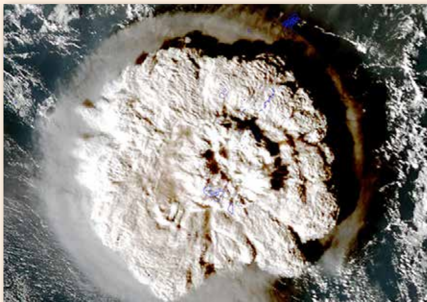
Εικόνα 7: Δορυφορική εικόνα που απεικονίζει την ηφαιστειακή έκρηξη του ηφαιστίου Hunga Tonga Hunga Ha'apai στις 15 Ιανουαρίου 2022. Τα νησιά του Βασιλείου της Τόνγκα παρουσιάζονται με το μπλε περίγραμμα (φωτογραφία από Tonga Geological Services).
