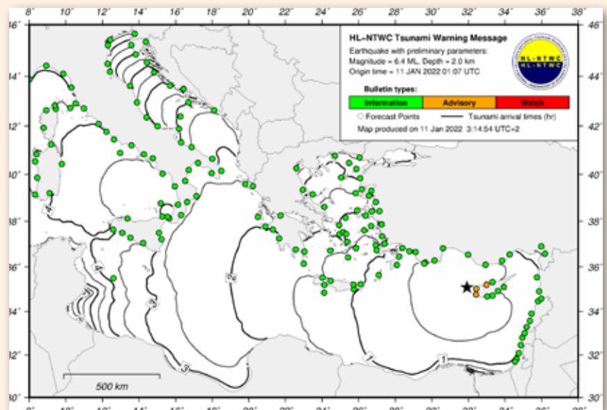
Εικόνα 5: Αυτοματοποιημένος χάρτης που λήφθηκε με το μήνυμα προειδοποίησης για τσουνάμι από το Εθνικό Κέντρο Προειδοποίησης για τσουνάμι του Γεωδυναμικού Ινστιτούτου του Εθνικού Αστεροσκοπείου Αθηνών, μετά από την εκδήλωση του πολύ ισχυρού σεισμού της 11 ης Ιανουαρίου 2022.
