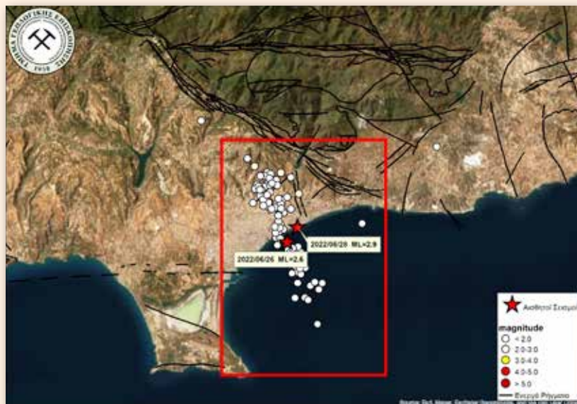
Εικόνα 6: Η σεισμική ακολουθία (σημνοσειρά) που καταγράφηκε στην Επαρχία Λεμεσού μεταξύ της 24 ης Ιουνίου 2022 και της 30 ης Ιουνίου 2022.
