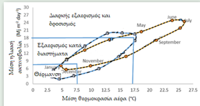
Σχήμα 1: Αναγκαίες παρεμβάσεις για τη δημιουργία κατάλληλου κλίματος στο εσωτερικό του θερμοκηπίου σε διαφορετικές τοποθεσίες. Η γραμμή με κόκκινο χρώμα αναφέρεται σε θερμοκήπιο τοποθετημένο σε μεσογειακές συνθήκες και η μπλε σε θερμοκήπιο τοποθετημένο σε ψυχρό κλίμα βορείων χωρών.
